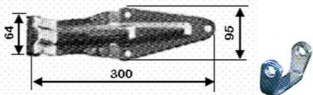
51 2061 Bagdørshængsel galv. 300x95x3 mm. 51 2062 Bagdørshængsel rustfri. 300x95x3 mm. 51 2071 Hængselryg galv., for 51 2061. Svejsbar. 51 2072 Hængselryg rustfri, for 51 2062. Svejsbar. 51 2082 Bolt rustfri, Ø12, for bgdørshængsler.
