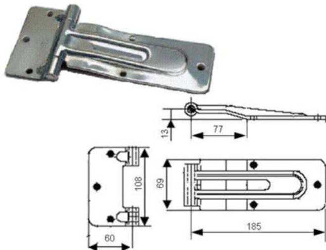
51 2056 Sidedørshængsel rustfri. 245x108 mm. Vægt 0,770 kg
