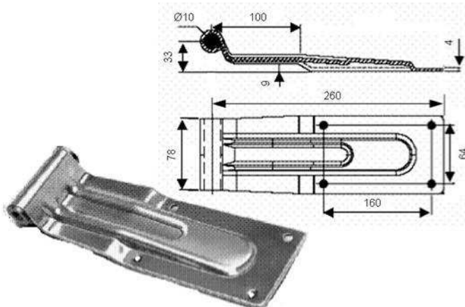
51 2012 Bagdørshængsel rustfri, 260x85 mm. Vægt 0,870 kg
