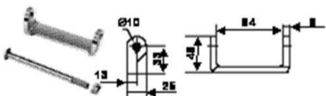
51 2026 Hængselryg m/bolt og møtrik rustfri. Svejsbar
