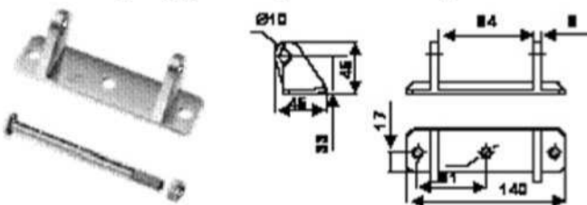
51 2024 Hængselryg m/bolt og møtrik rustfri. Skrå.
