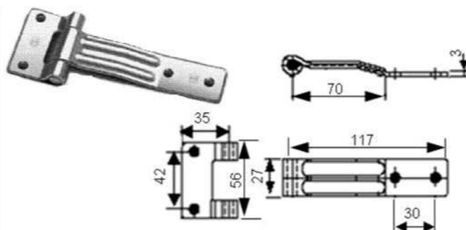
51 2044 Sidedørshængsel rustfri. 152x56 mm. Vægt 0,170 kg
