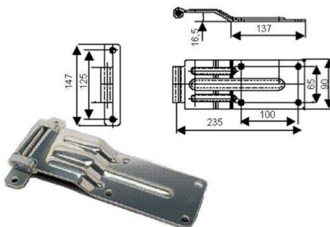
51 2034 Bagdørshængsel rustfri, dobbelt hængslet. Vægt 1,250 kg.
