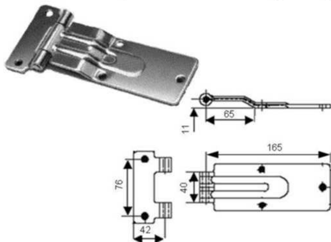
51 2054 Sidedørshængsel rustfri. 207x96 mm. Vægt 0,505 kg
