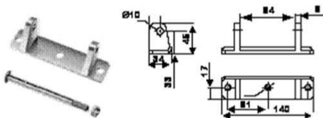
51 2022 Hængselryg m/bolt og møtrik rustfri. Lige.
