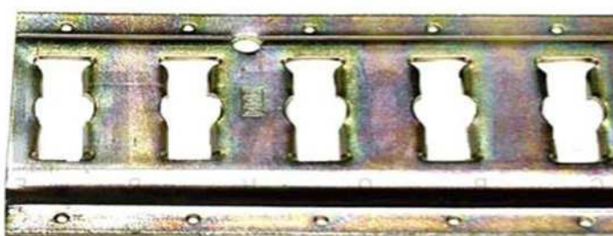
32 0536 Universalskinne, SØLV, m/drænhuller. Monteringshuller Ø5 mm. c/c 51 mm.. lgd.3000 mm. 32 0551 Endestykke i grå plast til universalskinner.
