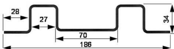
Tværsnit af skydestolpe
