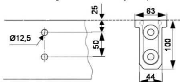
Montering af bundkasse for skydestolpe
